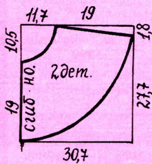
Деталь баски спинки
